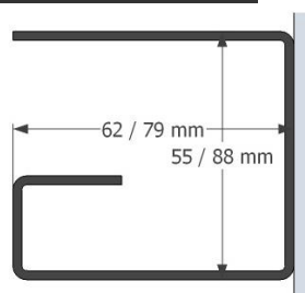
Guida con profilo a "G"
