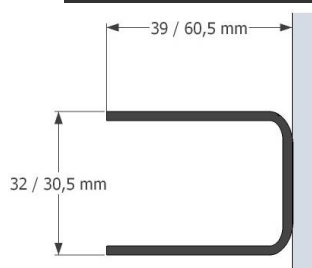
Guida classica ad "U"
